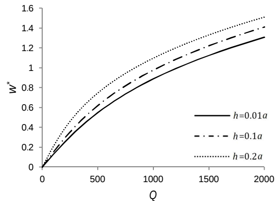
شکل 4 نمودار جابجایی عرضی بی‌بعد w^* بر حسب بار عرضی بی‌بعد Q برای ورق با تکیه‌گاه گیردار - گیردار
