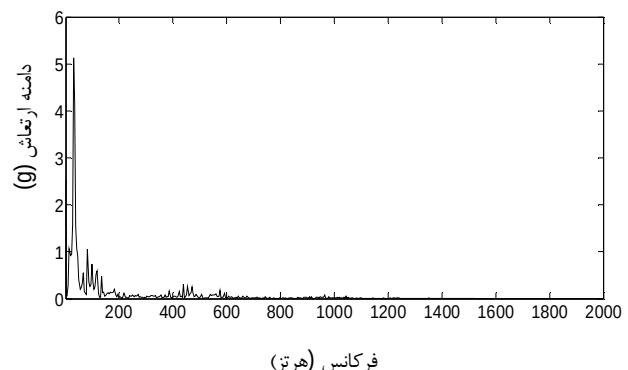
شکل 12 دامنه ارتعاش برای ابزار شکسته
