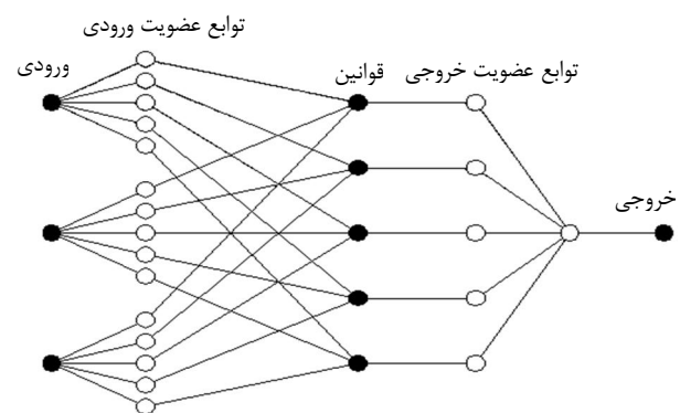
شکل 18 مدل انفیس پیشنهادی برای پایش وضعیت ابزار
