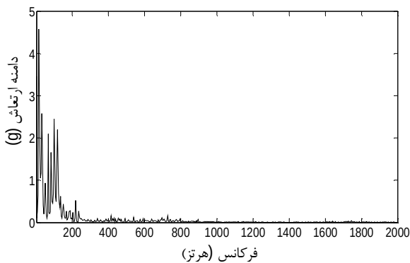
شکل 15 دامنه ارتعاش برای ابزار شکسته
