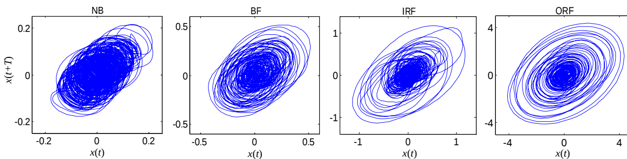
شکل 6 صفحه فاز بازسازی شده برای سیگنال‌های ارتعاشی بلبرینگ تحت بار سه اسب بخار
