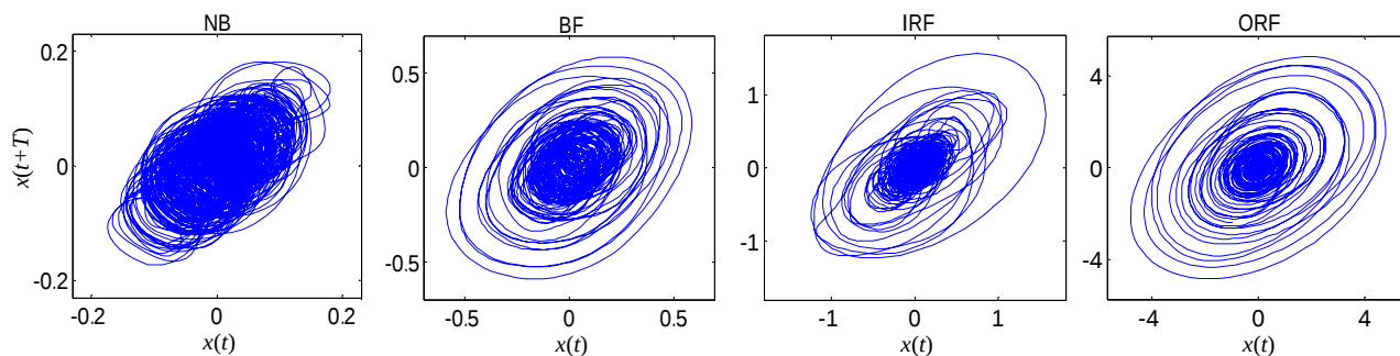
شکل 5 صفحه فاز بازسازی شده برای سیگنال‌های ارتعاشی بلبرینگ تحت بار دو اسب بخار
