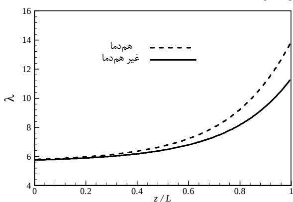
شکل 12 منحنی تغییرات محتوای آب در غشاء در دو حالت هم‌دم‌ها و غیر هم‌دم‌ها در چگالی جریان 1 \text{ A/cm}^2
