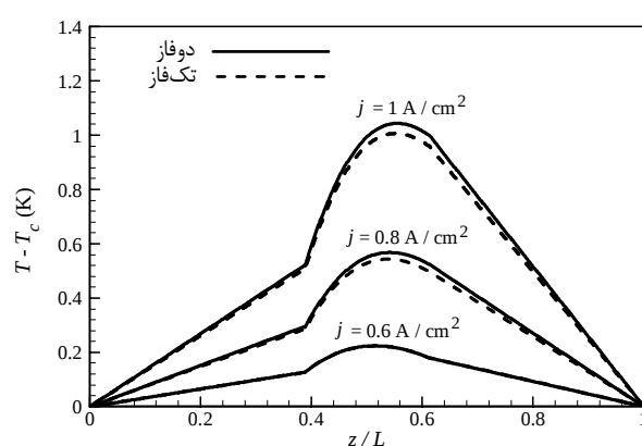
شکل 6 منحنی توزیع درجه حرارت در سراسر پیل سوختی به ازای چگالی جریان‌های مختلف در دو حالت تک‌فاز و دوفاز در رطوبت نسبی ورودی به کاتد 100%
