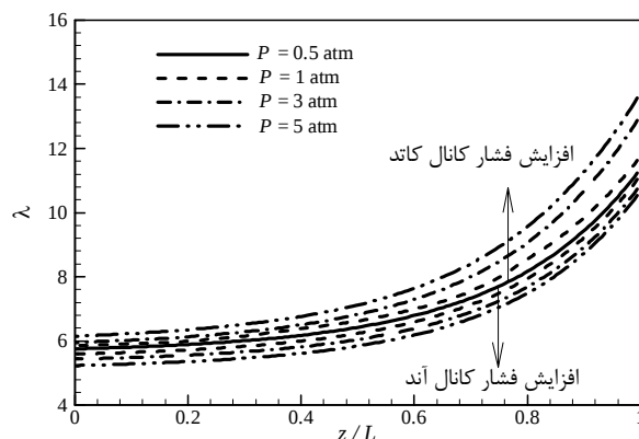
شکل 15 منحنی تغییرات محتوای آب غشاء به ازای فشار گاز ورودی به کاتد و آند متفاوت در چگالی جریان 1 \text{ A/cm}^2
