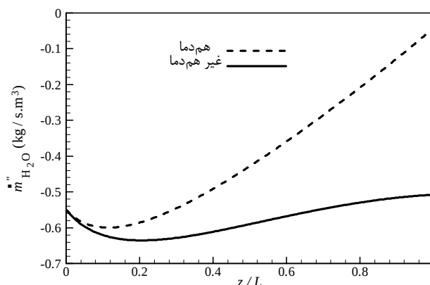
شکل 11 منحنی تغییرات نرخ تبخیر آب در طول لایه نفوذی گاز کاتد در دو حالت هم‌دم‌ها و غیر هم‌دم‌ها در چگالی جریان 1 \text{ A/cm}^2
