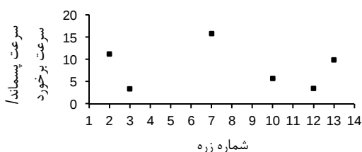
شکل 8 مقایسه نتایج سرعت برخورد - سرعت پسماند به صورت بی بعد برای زره های سوراخ شده
