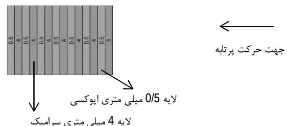
شکل 6 نمونه‌ای از لایه چینی مربوط به کد 7(4)C(0.5)E
