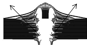
شکل 9 نحوه ایجاد تمرکز تنش و گسترش شکست مخروطی در زره کامپوزیت سرامیک - اپوکسی با لایه چینی 6(E1)C(4)
