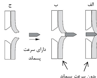
شکل 2 وضعیت‌های نهایی مختلف بعد از برخورد گلوله به زره: الف) ضبط گلوله ب) حد بالستیک ج) ایجاد سوراخ [1]
