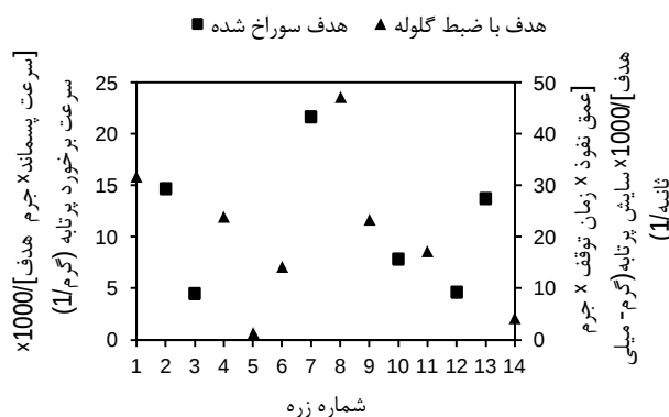
شکل 11 مقایسه کارایی بالستیک در هر دو هدف الف) هدف با ضبط گلوله با محور قایم سمت راست ب) هدف سوراخ شده با محور قایم سمت چپ
