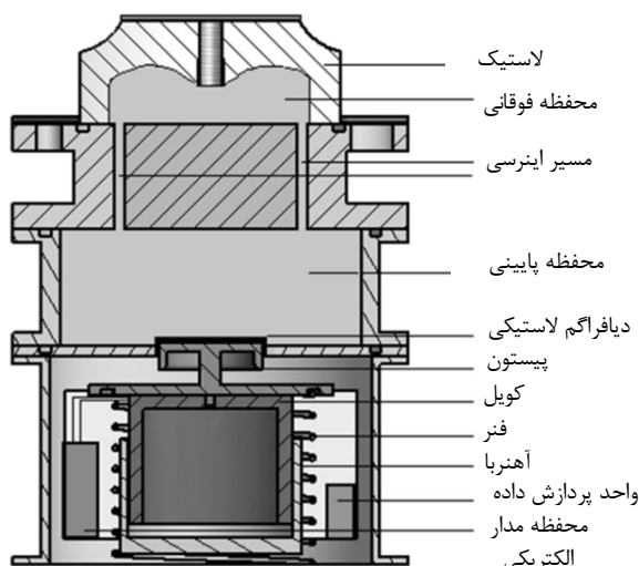
شکل 1 طراحی انجام شده برای دسته موتور هیدرولیکی فعال
