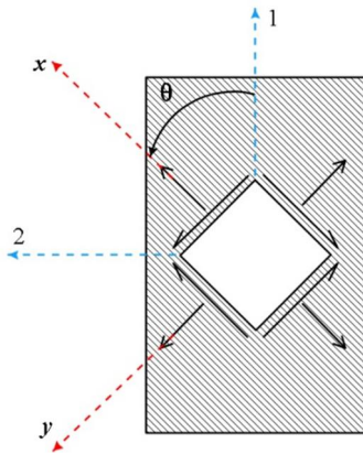
شکل 2 قرارداد جهات محوری و غیر محوری
