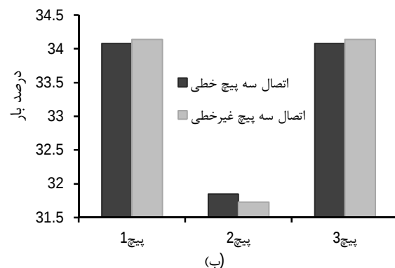
شکل 8 توزیع بار در اتصال تک‌لایه سه پیچ. الف - اتصال ا ب - اتصال II
