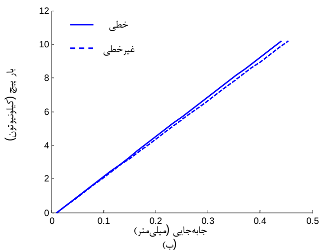
شکل 7 توزیع بار در اتصال تک‌لایه سه‌پیچه در حضور لقی؛ الف- در پیچ 2، ب- در پیچ 1 یا 3
