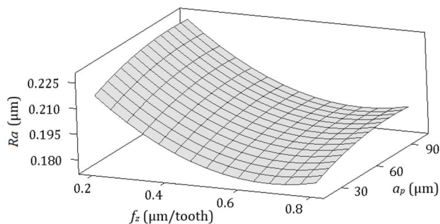
شکل 5 تأثیر پیشروی و عمق برش بر زبری سطح در شرایط نیمه‌خشک
