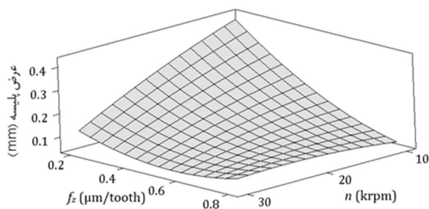
شکل 10 تأثیر سرعت اسپیندل و نرخ پیشروی بر عرض پلیسه در شرایط نیمه‌خشک
