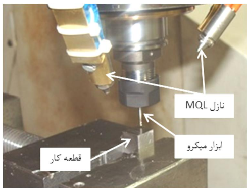
شکل 2 تجهیزات آزمایش‌های میکروفرزکاری شامل قطعه، نازل‌ها و ابزار برشی
