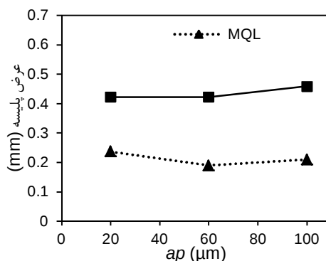
شکل 15 نمودار اثر عمق برش محوری بر عرض پلیسه
