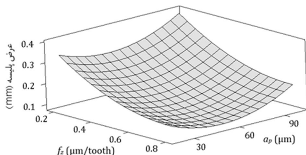
شکل 12 تأثیر نرخ پیشروی و عمق برش بر عرض پلیسه در شرایط نیمه‌خشک
