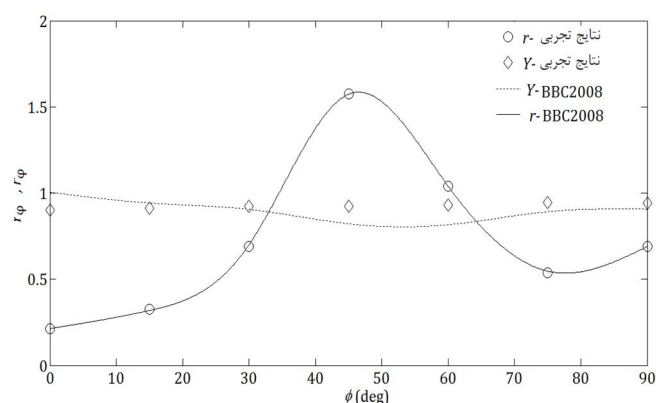
شکل 8 توزیع صفحه‌ای تنش تسلیم تک‌محوری و ضریب ناهمسانگردی پیش‌بینی
