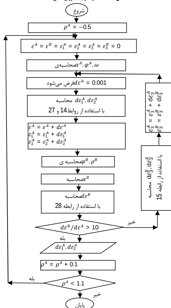
شکل 2 فلوجرات جهت تعیین کم نش‌های حدی بر اساس مدل MK
