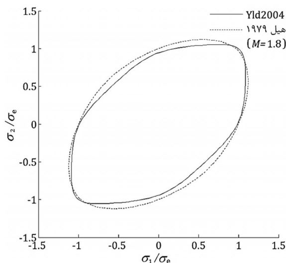
شکل 11 سطح تسلیم پیش‌بینی شده برای آلومینیوم AA6111-T4
