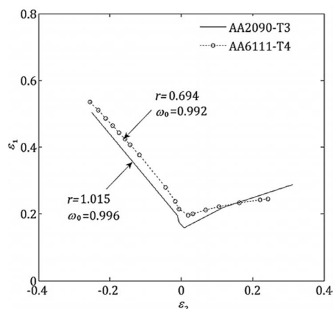
شکل 20 اثر ضریب ناهمسانگردی بر FLD براساس مدل MK و معیار تسلیم Yld2004
