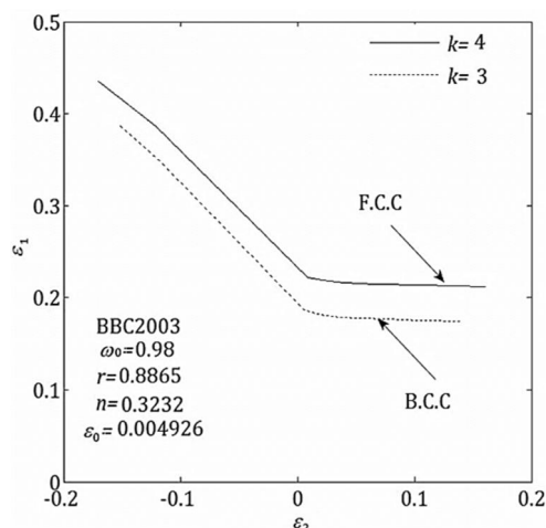
شکل 23 اثر توان معیار تسلیم بر FLD براساس مدل MK و معیار تسلیم BBC2003
