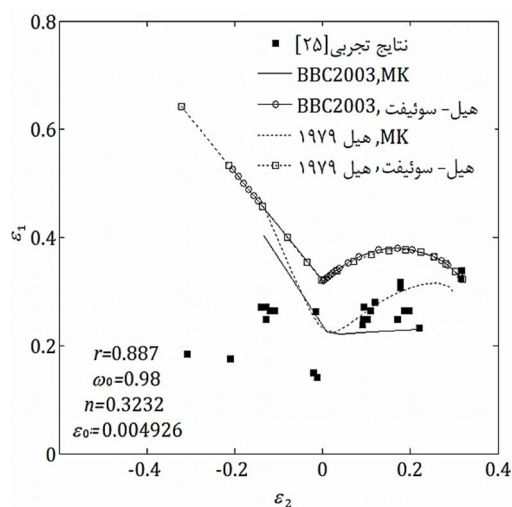
شکل 14 نمودار حد شکل‌دهی تجربی و پیش‌بینی شده برای آلیاژ AA5182-O
