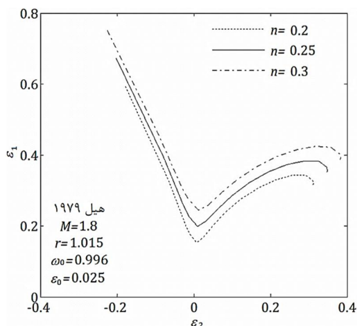
شکل 18 اثر توان کرنش‌سختی بر FLD براساس مدل MK و معیار تسلیم Hill 1979
