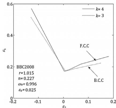
شکل 21 اثر توان معیار تسلیم بر FLD براساس مدل MK و معیار تسلیم BBC2008
