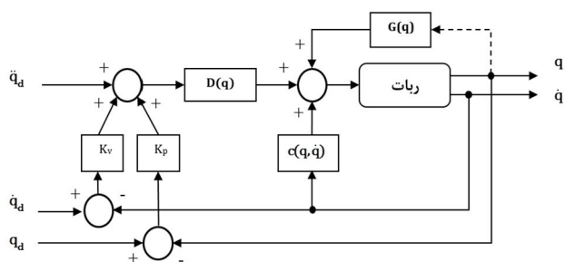
شکل 3 بلوک-دیاگرام CTC برای بازوی ماهر
