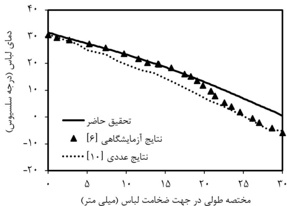
شکل 5 مقایسه نتایج مربوط به دما در تحقیق حاضر و نتایج عددی و آزمایشگاهی در آرایش ویسکوز-لیمینیت
