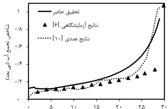
شکل 6 مقایسه نتایج مربوط به مقدار آب جمع شده در تحقیق حاضر و نتایج عددی و آزمایشگاهی در آرایش ویسکوز-لمینیت
