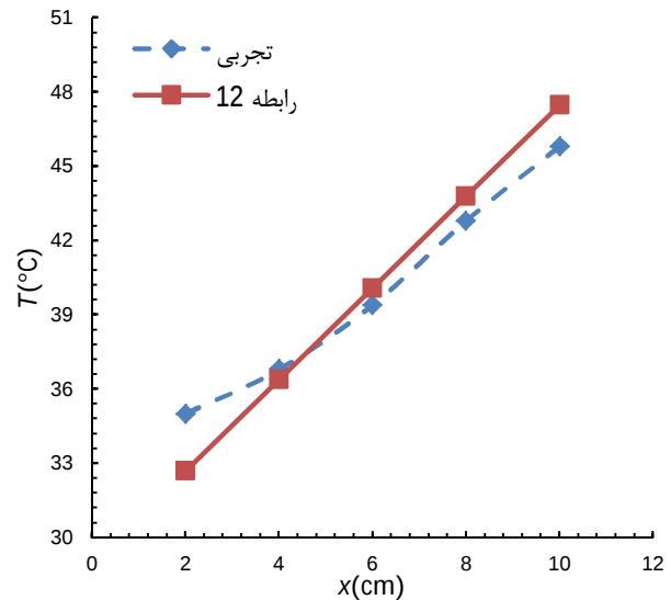
شکل 6 توزیع دمای سیال در طول کانال برای دانه‌بندی 5/5 میلی‌متر، به ازای نرخ جریان 140 لیتر بر دقیقه و در تولید حرارت 64/27 وات و مقایسه با رابطه تئوری
