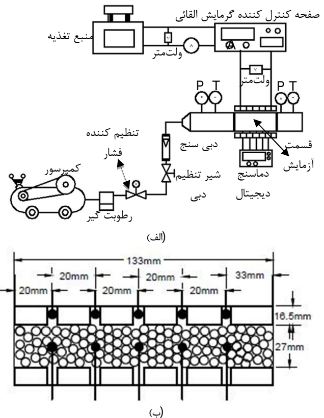
شکل 2 الف) شماتیک کلی دستگاه آزمایش ب) شماتیک قسمت آزمایش
