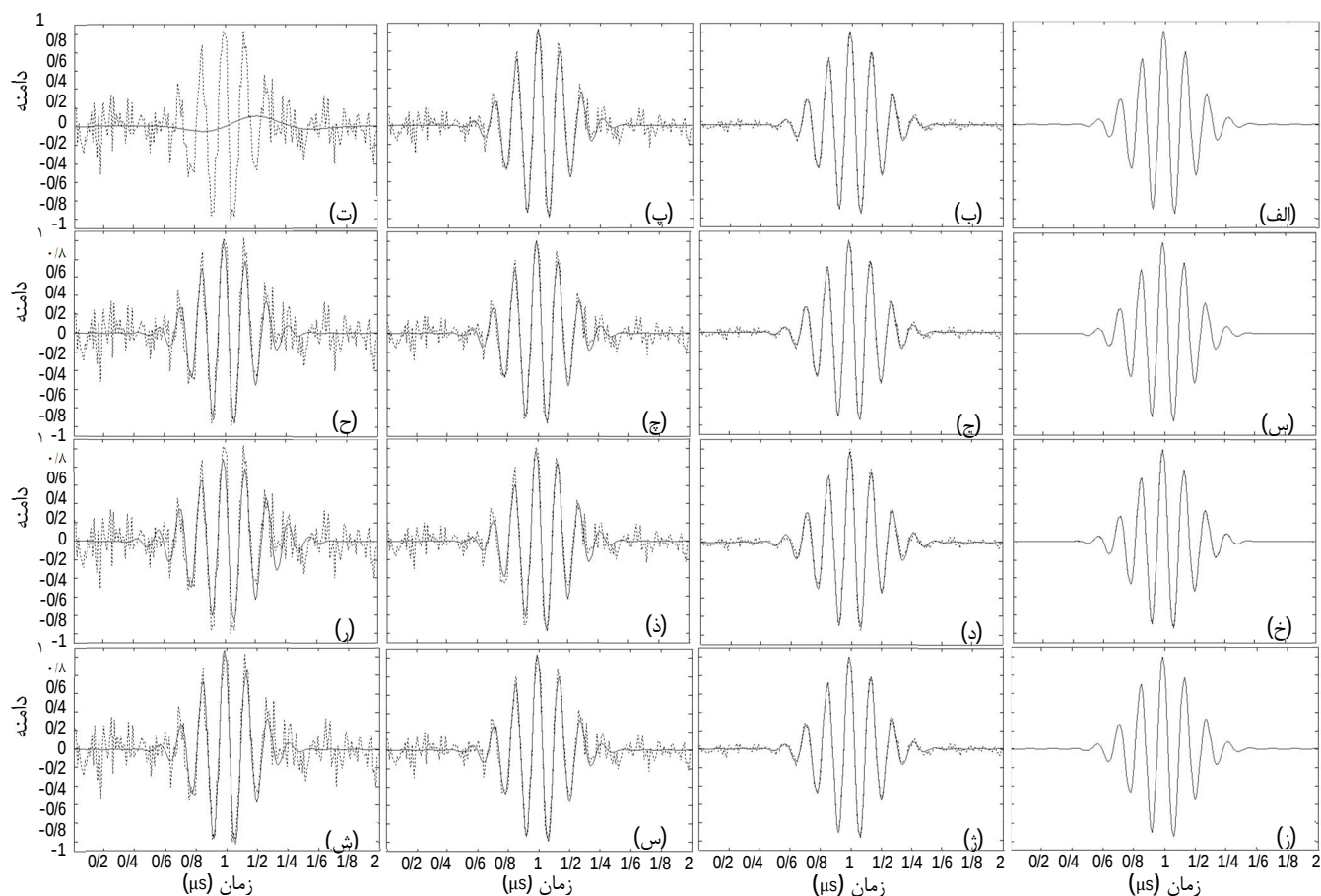
شکل 1 پژواک‌های شبیه‌سازی شده (خط چین) و اکوهای تخمین زده شده (خط ممتد). ستون اول، بدون نویز، ستون دوم، نسبت سیگنال به نویز ZVUB، ستون سوم، نسبت سیگنال به نویز 10dB، ستون چهارم، نسبت سیگنال به نویز 5dB. ردیف اول: گوس-نیوتن (الف تا ت)، ردیف دوم، بهینه‌سازی گروه ذرات (س تا ح)، ردیف سوم، الگوریتم ژنتیک (خ تا ر)، ردیف چهارم، الگوریتم ترکیبی بهینه‌سازی گروه ذرات و گوس-نیوتن (ز تا ش).
