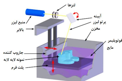
شکل 1 شمای کلی فرایند استریولیتوگرافی
