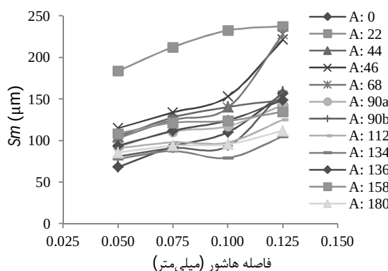
شکل 24 منحنی فاصله هاشور - Sm ، زمان بازپخت: 50 دقیقه، نمونه‌های D1, D2, D3, E1, E2, E3, F1, F2, F3
