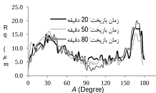
شکل 17 منحنی زاویه سطح - Rq، فاصله هاشورزنی: 0.100 mm
