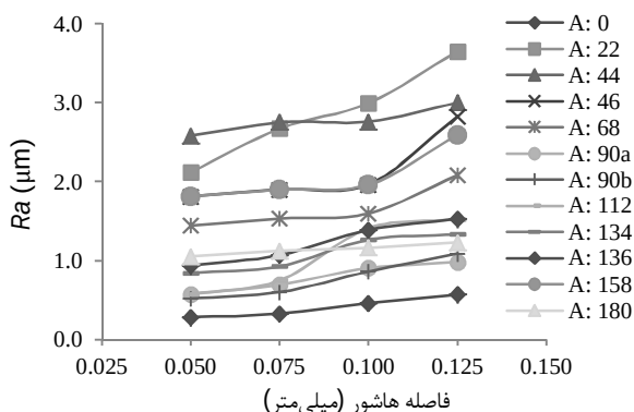
شکل 21 منحنی فاصله هاشور - Ra ، زمان بازپخت: 50 دقیقه، نمونه‌های D1, D2, D3, E1, E2, E3, F1, F2, F3
