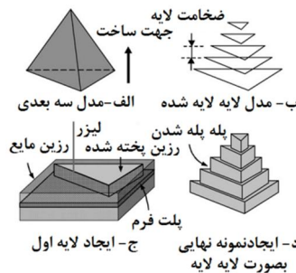
شکل 20 دلیل بروز پدیده پله پله شدن در فرایند استریلیتوگرافی [7]
