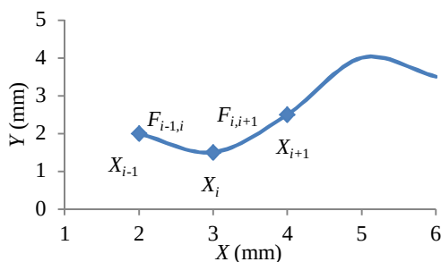
شکل 13 عبور دادن منحنی درجه سه از نقاط به‌دست آمده
