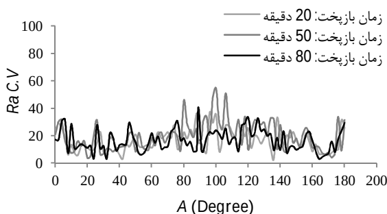
شکل 25 منحنی زاویه سطح- ضریب تغییرات Ra نمونه‌هایی با زمان بازپخت: 20، 50 و 80 دقیقه
