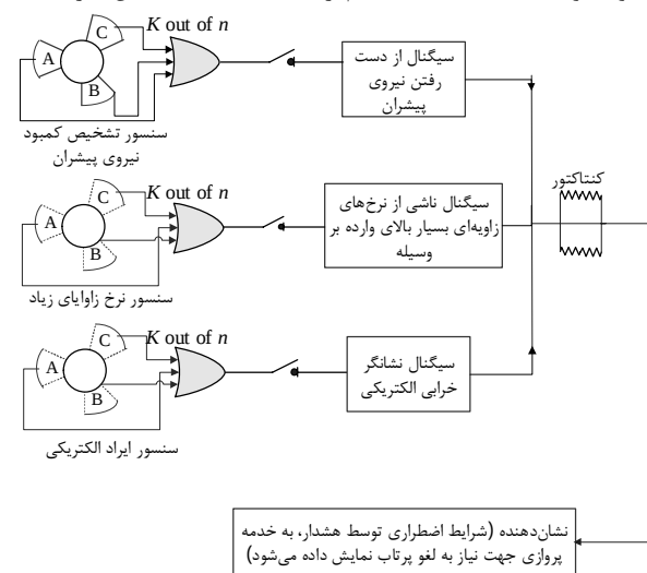
شکل 6 دیاگرام ساده‌سازی شده منسجم برای سیستم چندحالتی تشخیص شرایط اضطراری یک فضای
