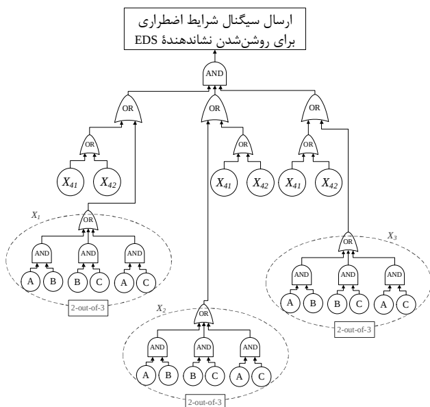
شکل 7 درخت خطای سیستم چندحالتی منسجم تشخیص شرایط اضطراری یک فضای
