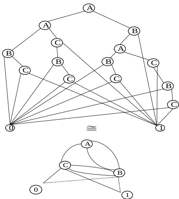
شکل 10 ساختار ROBDD برای درخت خطای بخش 2-out-of-3
