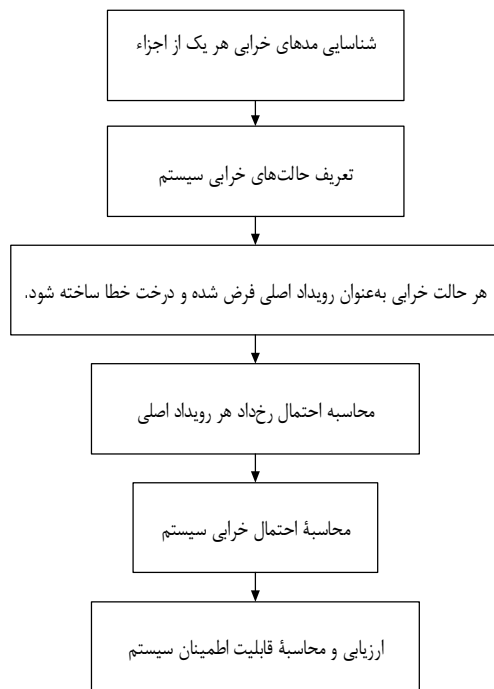
شکل 12 فلوچارت مربوط به آنالیز سیستم چندحالتی بر مبنای درخت خطا
