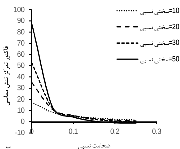
شکل 14 تغییرات فاکتور تمرکز تنش مماسی در راستای \theta = 90^\circ در فصل مشترک بتن سنگ در داخل بتن
