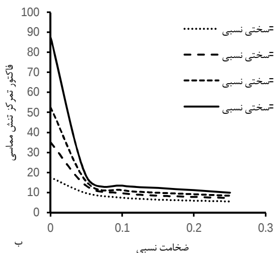
شکل 12 تغییرات فاکتور تمرکز تنش مماسی در راستای \theta = 90^\circ در مرز داخلی بتن
