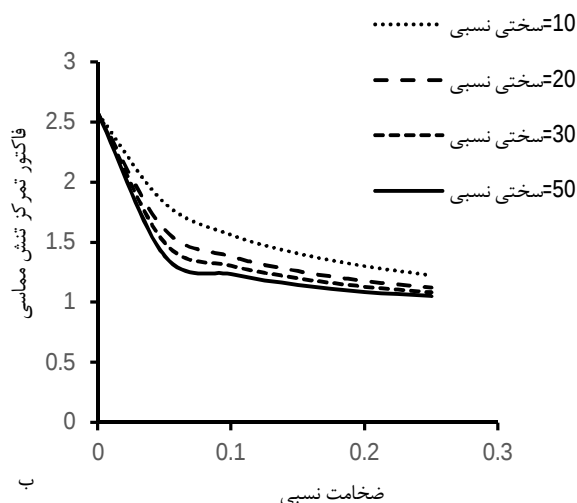
شکل 16 تغییرات فاکتور تمرکز تنش مماسی در راستای \theta = 90^\circ در فصل مشترک بتن سنگ در داخل سنگ
