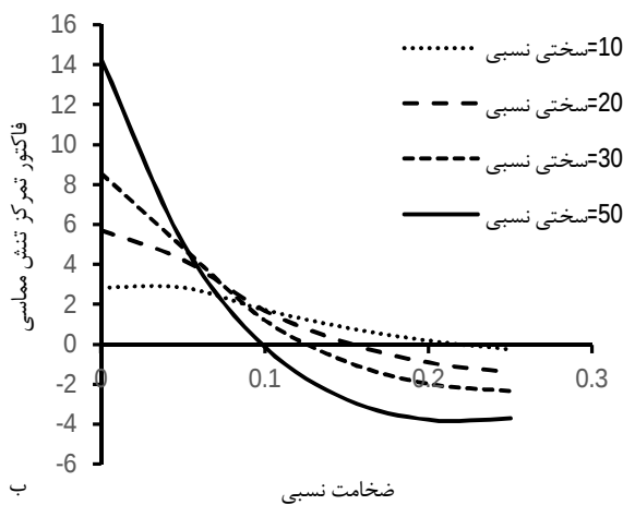
شکل 11 تغییرات فاکتور تمرکز تنش مماسی در راستای \theta = 0^\circ در مرز داخلی بتن
