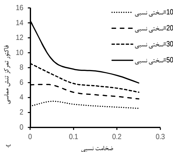
شکل 13 تغییرات فاکتور تمرکز تنش مماسی در راستای \theta = 0^\circ در فصل مشترک بتن سنگ در داخل بتن
