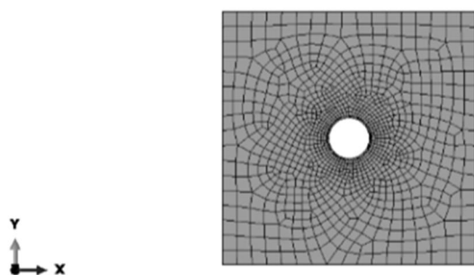
شکل 5 مدل‌سازی با نرم‌افزار المان محدود آباکوس
