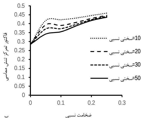
شکل 15 تغییرات فاکتور تمرکز تنش مماسی در راستای \theta = 0^\circ در فصل مشترک بتن سنگ در داخل سنگ
