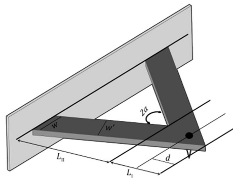
شکل 1 تیرک وی-شکل
