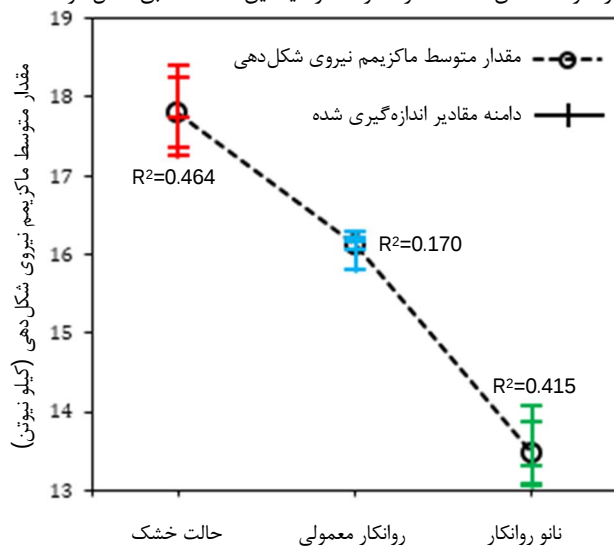
شکل 6 مقدار متوسط ماکزیم نیروی شکل‌دهی برای 5 بار تکرار آزمایش در هر شرایط روانکاری
