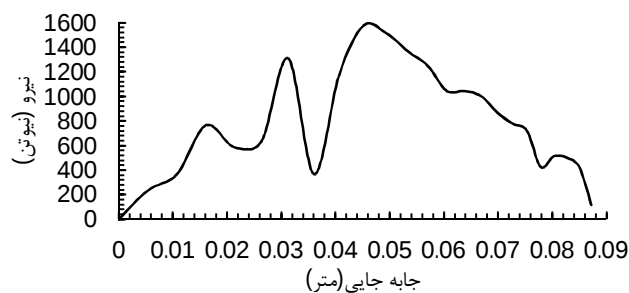
شکل 14 نمودار نیرو - جاب‌جایی نمونه مشبک 4
