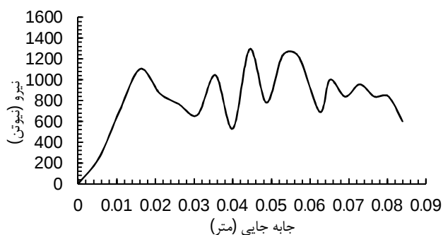
شکل 11 نمودار نیرو - جابه‌جایی نمونه مشبک 1
