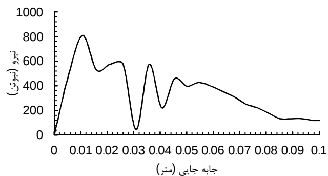
شکل 22 نمودار نیرو - جاب‌جایی نمونه مشبک 3-3
