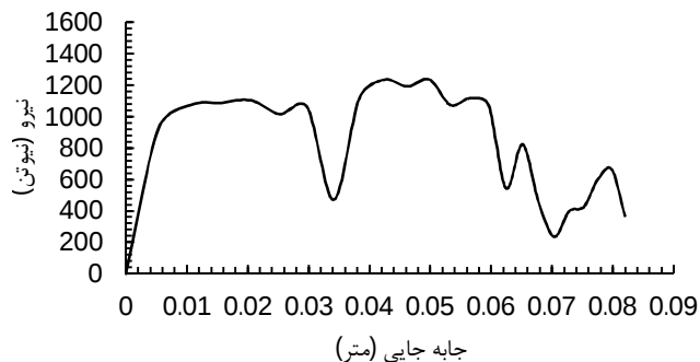
شکل 21 نمودار نیرو - جاب‌جایی نمونه مشبک 2-2
