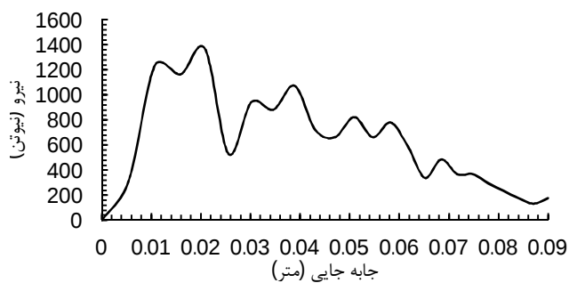
شکل 20 نمودار نیرو - جاب‌جایی نمونه مشبک 1-1
