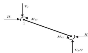
شکل 2 نیرو و گشتاور اعمال شده [3]
