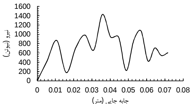
شکل 23 نمودار نیرو - جابه‌جایی نمونه مشبک 4-4
