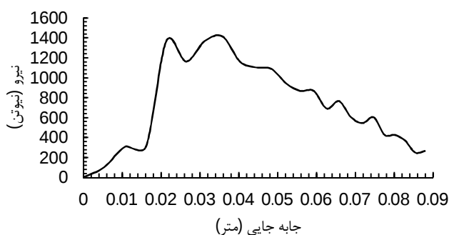
شکل 13 نمودار نیرو - جاب‌جایی نمونه مشبک 3
