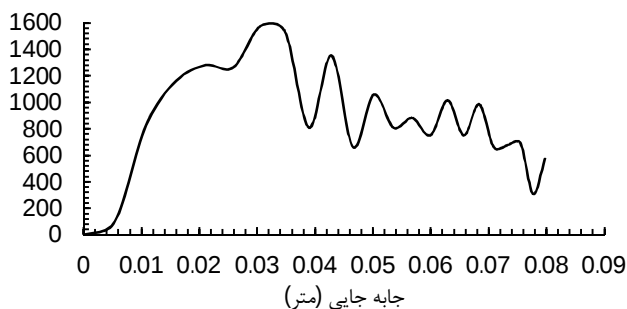
شکل 12 نمودار نیرو - جابه‌جایی نمونه مشبک 2
