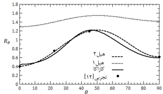
شکل 5 ضریب لانکفورد در آزمون کشش تک‌محوره با زاویه \theta نسبت به جهت نورد ورق در دمای اتاق
