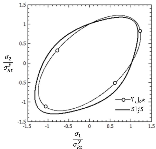
شکل 4 مقایسه سطح تسلیم کازاکا و هیل در حالت تنش دومحوره آلیاژ تیتانیوم در دمای 400^\circ\text{C}
