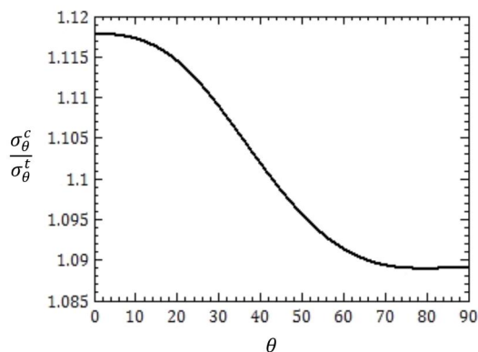
شکل 9 نسبت تنش تسلیم فشاری به کششی در آزمون تک‌محوره با زاویه \theta نسبت به جهت نورد ورق به تنش تسلیم در جهت نورد ورق در دمای 400^\circ\text{C} (سطح تسلیم کازاکا)
