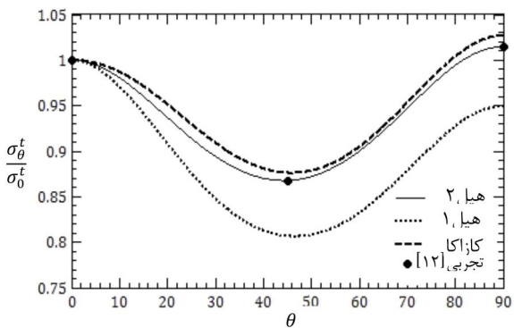
شکل 8 نسبت تنش تسلیم در آزمون کشش تک‌محوره با زاویه \theta نسبت به جهت نورد ورق به تنش تسلیم در جهت نورد ورق در دمای 400^\circ\text{C}
