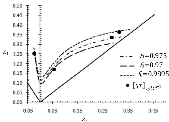
شکل 10 تأثیر پارامتر f_0 در پیش بینی حد شکل دهی ورق تیتانیوم در دمای 400°C و سطح تسلیم کازاکا
