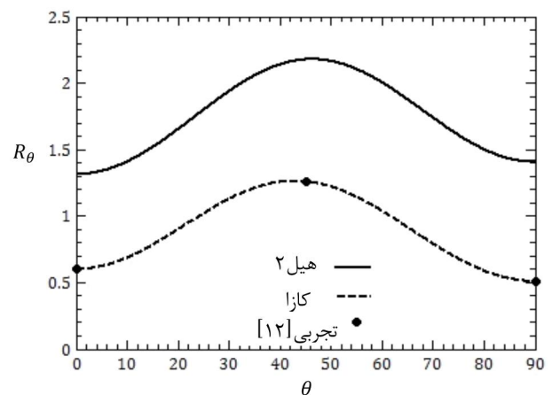
شکل 6 ضریب لانکفورد در آزمون کشش تک‌محوره با زاویه \theta نسبت به جهت نورد ورق در دمای 400^\circ\text{C}
