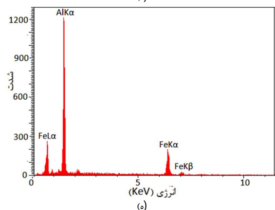
شکل 3 فصل مشترک اتصال صفحات آلومینیوم و فولاد پس از عملیات حرارتی در دمای 350 درجه سانتی گراد و مدت 6 ساعت (الف) تصویر میکروسکوپ الکترونی (ب) آنالیز شیمیایی خطی فصل مشترک اتصال (ج) آنالیز EDS نقطه 1 نشان داده شده در شکل 3-الف (د) آنالیز EDS نقطه 2 نشان داده شده در شکل 3-الف (ه) آنالیز EDS نقطه 3 نشان داده شده در شکل 3-الف
