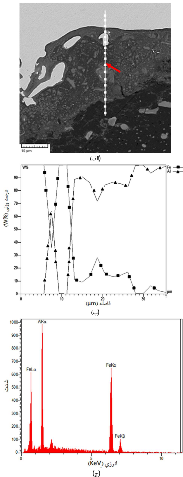
شکل 2 فصل مشترک اتصال صفحات آلومینیوم و فولاد پس از عملیات حرارتی در دمای 300 درجه سانتیگراد و مدت 60 دقیقه (الف) تصویر میکروسکوپ الکترونی (ب) آنالیز شیمیایی خطی فصل مشترک اتصال (ج) آنالیز EDS نقطه نشان داده شده در شکل 2- الف
