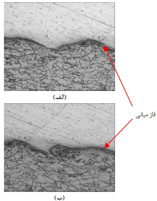
شکل 1 فصل مشترک نمونه جوش انفجاری شده (الف) فصل مشترک بالا (ب) فصل مشترک پایین
