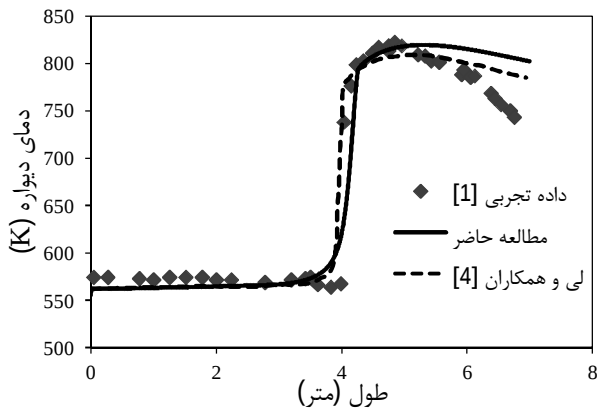
شکل 11 توزیع دمای دیواره کانال و افزایش ناگهانی آن
