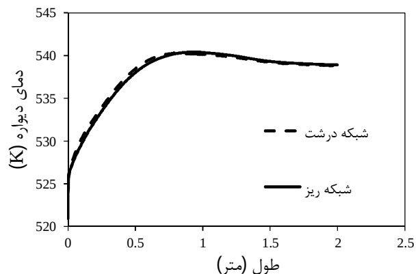
شکل 5 توزیع دمای دیواره در راستای طول کانال با شبکه‌های مختلف
