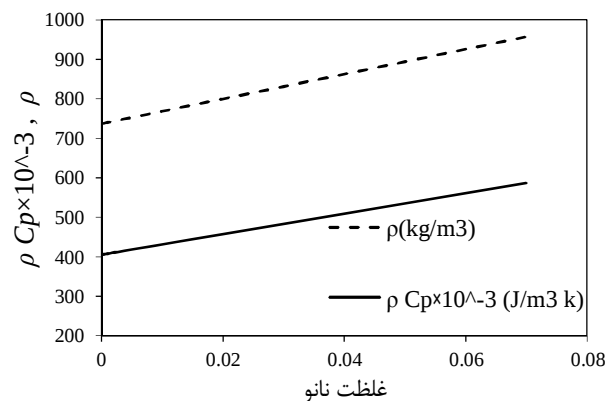
شکل 2 تغییرات چگالی و حاصل ضرب چگالی در ظرفیت گرمایی ویژه برای غلظت‌های مختلف نانوذره
