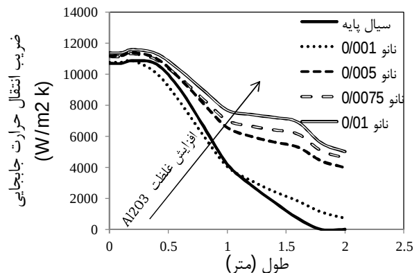
شکل 14 ضریب انتقال حرارت جابجایی فاز مایع با غلظت‌های مختلف نانوذره
