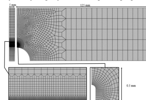
شکل 5 نمایش مش‌بندی مدل سه‌بعدی SEN(B) و المان‌های نزدیک به نوک ترک
