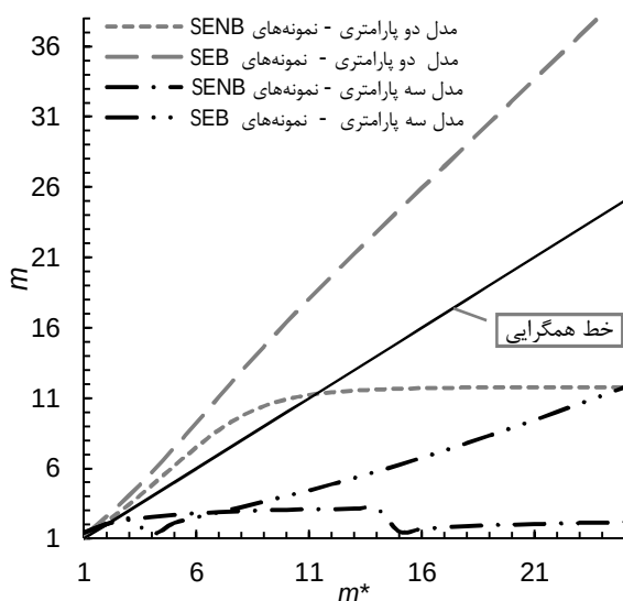
شکل 8 نتایج حاصل از کالیبراسیون پارامترهای رویکرد موضعی در نمونه‌های SEN(B) و SEN(B) از طریق مدل‌های دو پارامتری و سه پارامتری با استفاده از روش تطبیق پارامتر شکل ویبال ( m )
