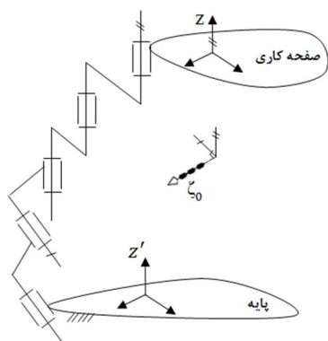
شکل 5 نمایش، یای \bar{R}\bar{R}\bar{R}\bar{R}\bar{R} از بازوی 3T1R
