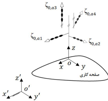
شکل 8 وضعیت هندسی رنج‌های تحریک با شرایط m_{ai}^T r_a = 0 ( i = 1, 2, 3 ) و m_{a4}^T r_a \neq 0
