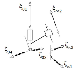
شکل 2 سیستم توئیست متقابل با سیستم رنج (\zeta_0 - 2) - سیستمی
