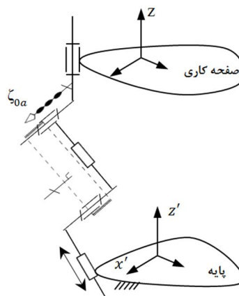
شکل 9 نمایش رنج تحریک موثر گام صفر با محور ثابت از پای
