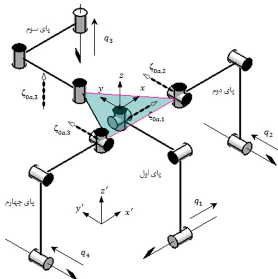
شکل 10 بازوی P(RRR)_E \parallel \hat{R}, 2P(RRR)_E \parallel \hat{R}, P(RRR)_E \parallel \hat{R} از گروه (x)(z)(y, \alpha) با نمایش محور رنج تحریک
