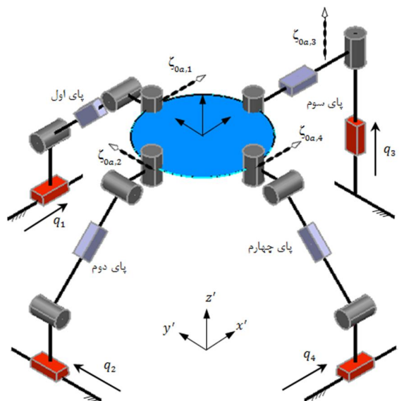
شکل 11 بازوی P(RRR)_E \parallel \hat{R}, P(RPR)_E \parallel \hat{R}, P(RPR)_E \parallel \hat{R} از گروه (z)(x)(y, \alpha) با نمایش محور رنج تحریک
