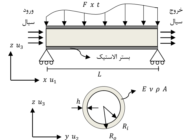
شکل 1 تصویری از نانولوله مورد مطالعه و ویژگی های مکانیکی و هندسی آن
