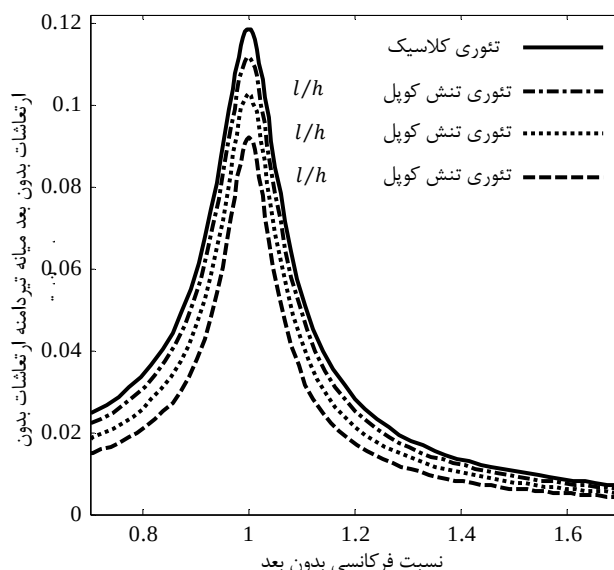
شکل 2 پاسخ فرکانسی سیستم به ازای مقیاس‌های طول متفاوت در تئوری تنش کوپل و در تئوری کلاسیک
