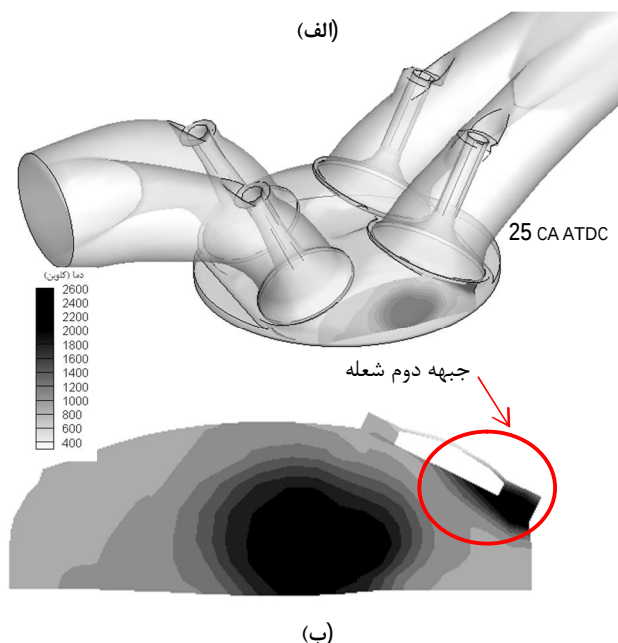
شکل 12 شکل شعله در منسعی (ب)، عرضی و ب: طولی از سیلندر
