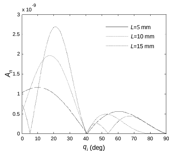
شکل 7 نمودار ضریب دامنه مود M3 در اتصال چسبی سه لایه آلومینیوم-اپوکسی-آلومینیوم برای یک منبع با ابعاد محدود برحسب پارامترهای ترنسیدوسر تابش در فرکانس 0/25 MHz
