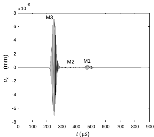
شکل 10 نمودار جابجایی درون صفحه‌ای برحسب زمان در فاصله 1m از مبدا مختصات بر روی سطح بالایی اتصال چسبی سه لایه
