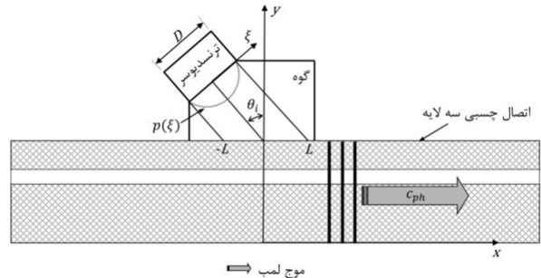
شکل 2 مدل تولید موج لمب توسط ترنسیدوسر تابش زاویه‌ای
