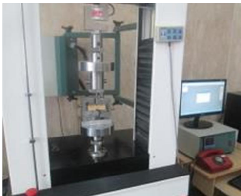
شکل 8 دستگاه آزمایش فشار الکترومکانیکی سنتم
