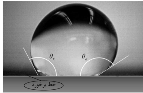
شکل 2 زوایای پیش‌رو و پس‌رو در برخورد قطره با سطح جامد
