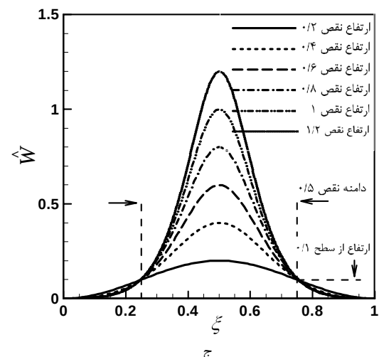
شکل 2 تغییر دامنه، مکان و ارتفاع نقص در تحلیل آیرودلاستیک صفحه
