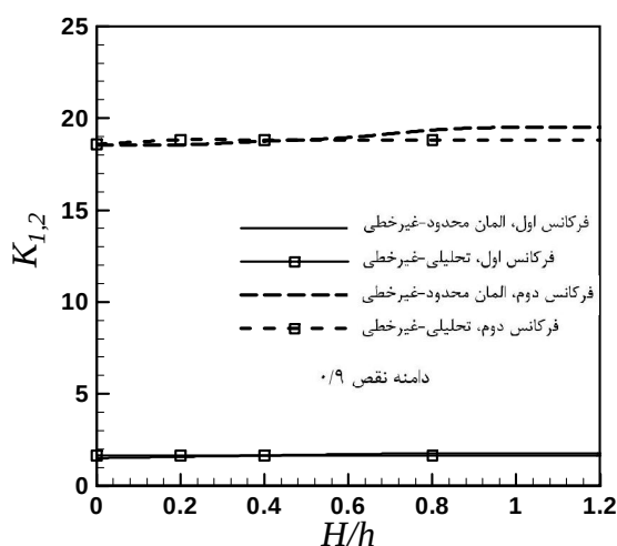
ب مقایسه تغییرات فرکانس سازه با اثر نقص کوچک به روش تحلیلی و المان محدود
