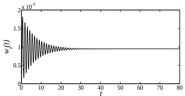
شکل 6 جابجایی نوک تیر با سطح مقطع غیر یکنواخت در حالتی که میرایی مودال سیستم از مقدار بحرانی بیشتر است ( \xi = 0.03 , \bar{U} = 10 \text{ m/s} )
