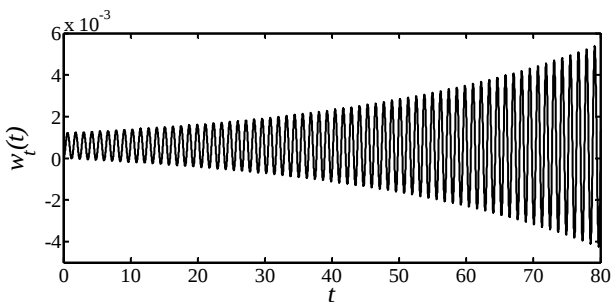
شکل 7 جابجایی نوک تیر با سطح مقطع غیریکنواخت در حالتی که میرایی مودال سیستم از مقدار بحرانی کم‌تر است ( \xi = 0.005 , \bar{U} = 80 \text{ m/s} )
