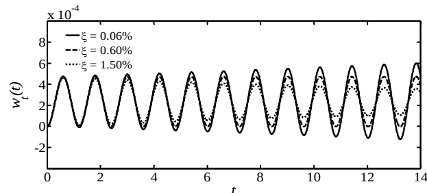
شکل 8 تأثیر میرایی بر جابجایی نوک تیر با مقطع غیریکنواخت ( \bar{U} = 50 \text{ m/s} )
