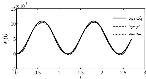
شکل 5 تأثیر افزایش تعداد شکل مودها در تخمین پاسخ دینامیکی
