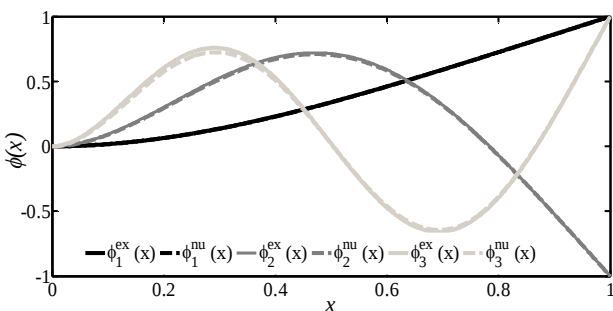
شکل 2 شکل مودهای تیر یکنواخت، مقایسه نتایج حل عددی و حل دقیق
