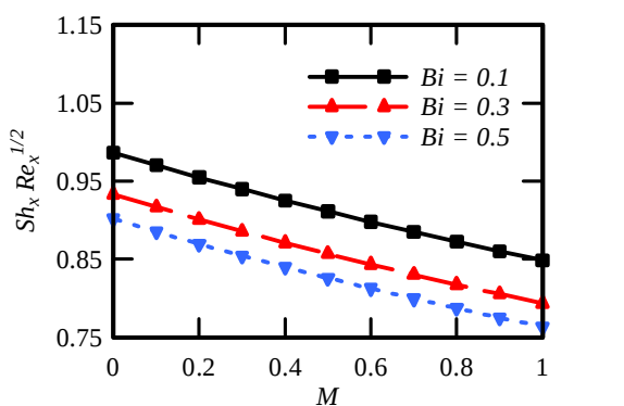
شکل 12 تأثیر عدد بیوت به ازای مقادیر مختلف پارامتر مغناطیسی و Nb = Nt = 0.1 , Pr = 0.71 , Le = 2 , \gamma = 0.25 و \lambda = 0.5
