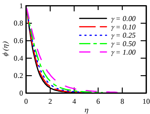
شکل 7 تأثیر پارامتر سرعت لغزشی به ازای M = 1, Nb = Nt = 0.1 Bi = 0.1 و \lambda = 0.5, Le = 2, Pr = 0.71
