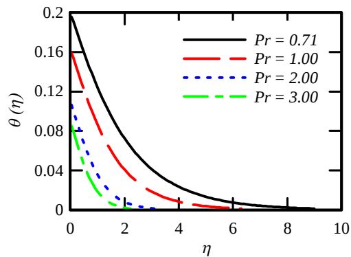
شکل 4 تأثیر عدد پراکتل بر توزیع دما به ازای Le = Nb = Nt = 0.1, M = 1 Bi = 0.1 و \lambda = 0.5, \gamma = 0.25, 2
