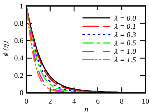
شکل 8 تأثیر پارامتر نسبت نرخ کشش به ازای M = 1 , Nb = Nt = 0.1 , Pr = 0.71 , Bi = 0.1 و \gamma = 0.25 , Le = 2
