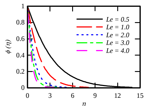
شکل 5 تأثیر عدد لوییس بر توزیع غلظت به ازای M = 1, Nb = Nt = 0.1 Bi = 0.1 و \lambda = 0.5, \gamma = 0.25, Pr = 0.71
