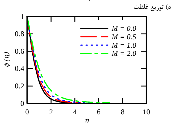
شکل 3 تأثیر پارامتر مغناطیسی به ازای Le = Pr = 0.71 , Nb = Nt = 0.1 و Bi = 0.1 و \lambda = 0.5 ، \gamma = 0.25 ، 2
