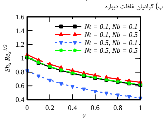
شکل 11 تأثیر پارامترهای حرکت براونی و انتشار حرارتی به ازای مقادیر مختلف پارامتر سرعت لغزشی و M = 1 , Pr = 0.71 , Le = 2 , \lambda = 0.5 و Bi = 0.1
