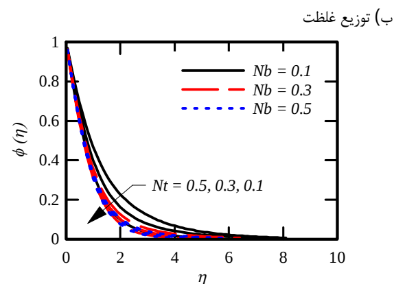
شکل 6 تأثیر پارامتر حرکت براونی و پارامتر انتشار حرارتی به ازای M = 1 Bi = 0.1 و \lambda = 0.5, \gamma = 0.25, Le = 2, Pr = 0.71
