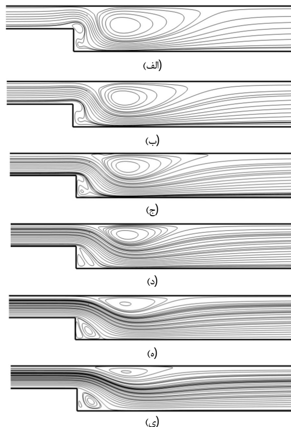
شکل 12 تاثیر عدد رینولدز بر جریان سیال V=18 \text{ kV} , \alpha = 45^\circ (الف) \text{Re}=770 (ب) \text{Re}=1050 (ج) \text{Re}=1330 (د) \text{Re}=1610 (ه) \text{Re}=1890 (و) \text{Re}=2170
