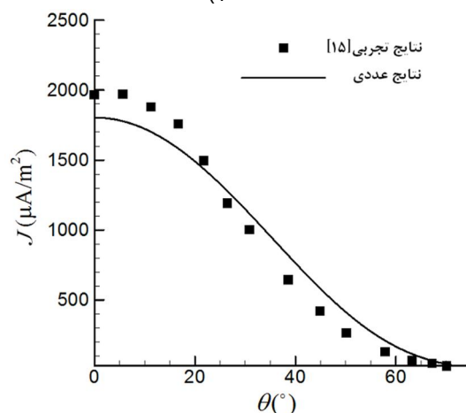
شکل 6 مقایسه توزیع چگالی جریان الکتریکی حاصل از تحلیل عددی و نتایج تجربی (V = 18 \text{ kV})
