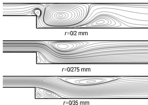
شکل 11 خطوط جریان در شعاع‌های مختلف الکتروود تزریق‌کننده ( \alpha = 45^\circ, V = 18 \text{ kV}, Re = 530 )
