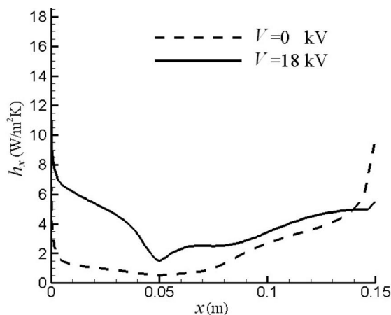
شکل 13 ضریب انتقال حرارت موضعی ( \alpha = 45^\circ , \text{Re}=770 )
