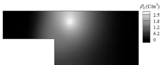
شکل 8 توزیع چگالی بار الکتریکی V=18 \text{ kV} , \alpha = 45^\circ
