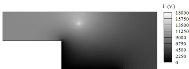
شکل 7 توزیع پتانسیل الکتریکی V=18 \text{ kV} , \alpha = 45^\circ
