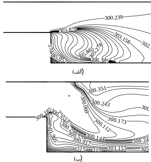
شکل 10 خطوط هم دما ( \alpha = 45^\circ ) الف) V=0 \text{ kV} ب) V=18 \text{ kV}
