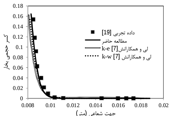
شکل 8 توزیع کسر حجمی بخار در فاصله 0/816 متر از مقطع خروجی
