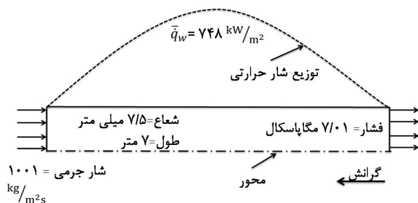
شکل 9 شماتیکی از هندسه مساله به همراه شرایط مرزی
