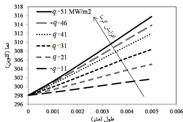
شکل 18: توزیع دمای توده سیال مایع در امتداد مینی کانال با شار گرمایی اعمالی مختلف
