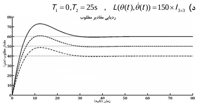
شکل 13 ردیابی مقادیر مطلوب - ضریب مشاهده‌گر اغتشاش بزرگ
