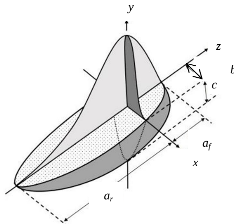
شکل 5 مدل منبع حرارتی حجمی دوبیضی‌گون گلدک [14]
