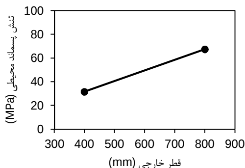
شکل 15 اثر قطر خارجی بر روی بیشینه تنش پسماند محیطی
