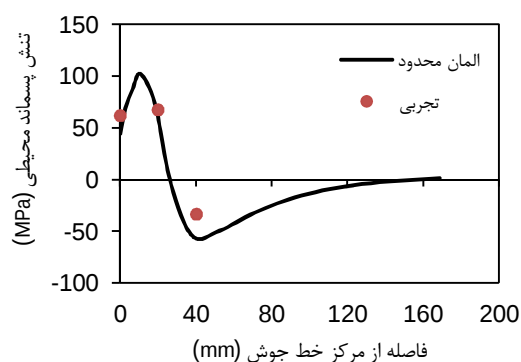
شکل 12 مقایسه تنش‌های پسماند ناشی از المان محدود با نتایج تجربی الف. تنش پسماند محوری ب. تنش پسماند محیطی
