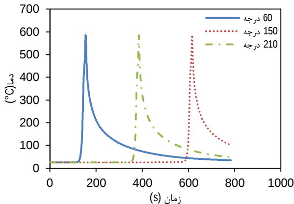
شکل 7 چرخه حرارتی جوش در فاصله 5 میلی‌متری از مرکز خط جوش بر روی مقاطع مختلف از شروع جوش
