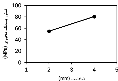
شکل 20 اثر ضخامت بر روی بیشینه تنش پسماند محوری
