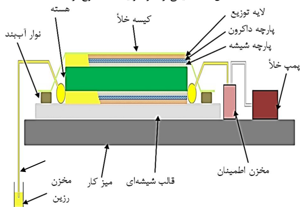
شکل 3 شماتیک فرآیند انتقال رزین به کمک خلأ
