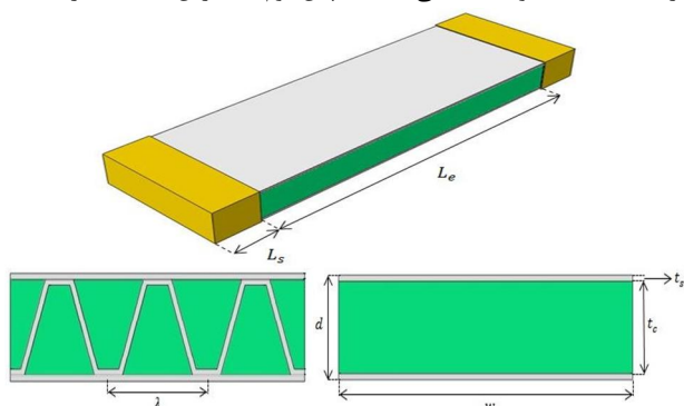
شکل 1 شماتیک نمونه، مقطع نمونه با هسته ساده و مقطع نمونه با هسته موج‌دار
