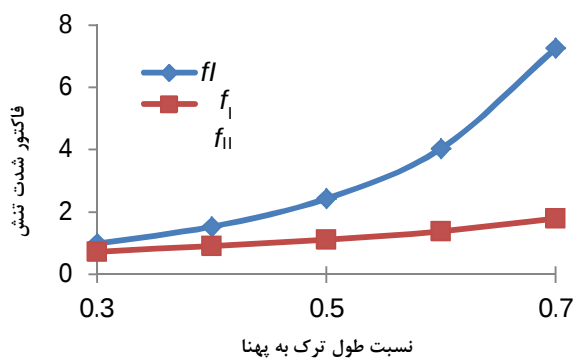
شکل 8 نمودار تغییر ضرایب تصحیح هندسی برحسب نسبت طول ترک به پهناي نمونه
