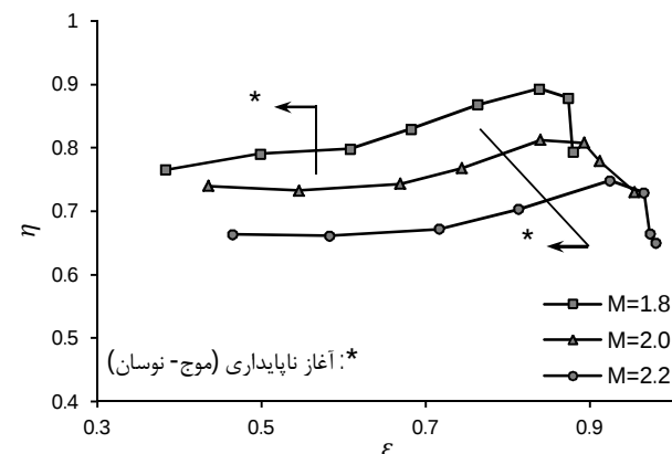
شکل 5 نمودار عملکردی ورودی در اعداد ماخ 1/8، 2/0 و 2/2
