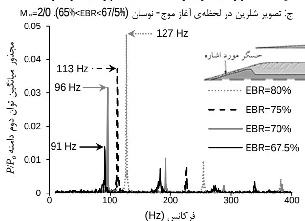
شکل 7 نمودار پاسخ فرکانسی یکی از حسگرهای فشار استاتیک دماغه در M_{\infty}=2/0
