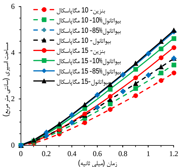
شکل 14 مقایسه مساحت پاشش سوخت های مورد بررسی با افزایش فشار تزریق از 10 مگاپاسکال به 15 مگاپاسکال
