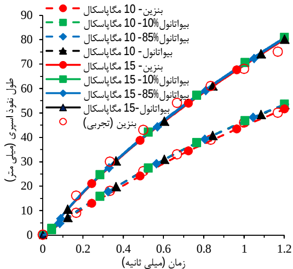
شکل 13 مقایسه طول نفوذ سوخت های مورد بررسی با افزایش فشار تزریق از 10 مگاپاسکال به 15 مگاپاسکال
