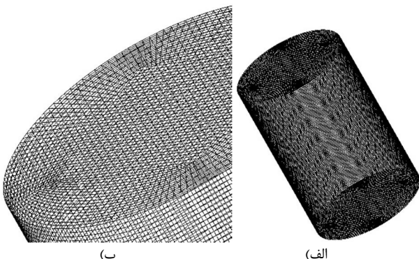
شکل 2 الف) قلمرو محاسباتی ب) نمایی دقیق تر از قلمرو محاسباتی
