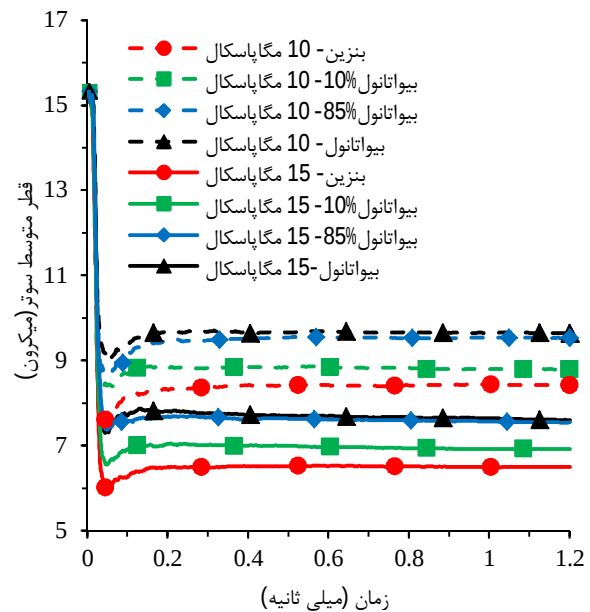
شکل 15 مقایسه ی قطر متوسط سوتر سوخت های مورد بررسی با افزایش فشار تزریق از 10 مگاپاسکال به 15 مگاپاسکال
