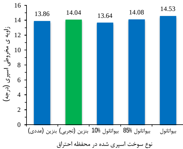
شکل 6 زاویه ی مخروط سوخت های مختلف در فشار محیط 600 کیلو پاسکال و فشار تزریق 10 مگا پاسکال
