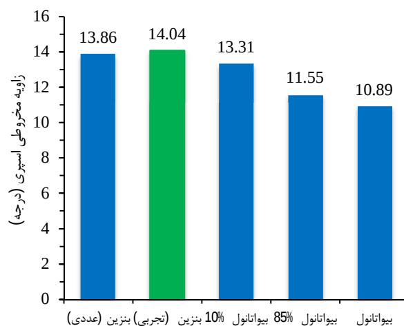
شکل 17 زاویه مخروط سوخت‌های مختلف با ثابت ماندن انرژی سوخت تزریق شده و مدت زمان پاشش
