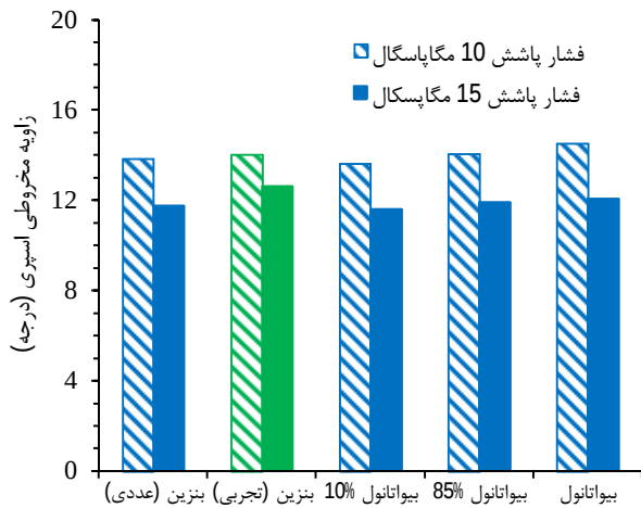
شکل 12 مقایسه زاویه مخروط سوخت های مورد بررسی با افزایش فشار تزریق از 10 مگاپاسکال به 15 مگاپاسکال
