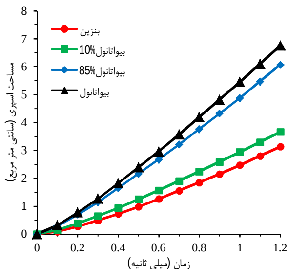
شکل 19 مساحت پاشش سوخت‌های مورد بررسی با ثابت ماندن انرژی سوخت تزریق شده و مدت زمان پاشش
