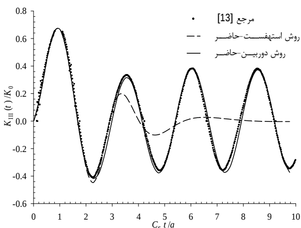
شکل 5 ضریب شدت تنش دینامیکی بی بعد، K_{III}(t)/K_0 ، بر حسب زمان بی بعد، C_s t/a در صفحه بی نهایت تحت بار هارمونیک با عدد موج \varpi = 2.5 .
