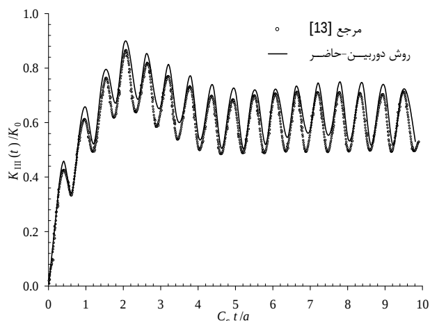
شکل 7 ضریب شدت تنش دینامیکی بی‌بعد، K_{III}(t)/K_0 ، بر حسب زمان بی‌بعد، C_s t/a ، در صفحه بی‌نهایت تحت بار نوسانی با عدد موج \varpi = 4.5 .
