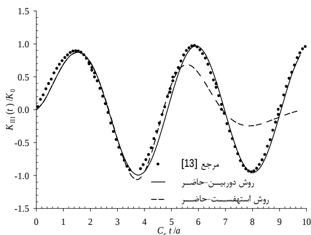
شکل 4 ضریب شدت تنش دینامیکی بی بعد، K_{III}(t)/K_0 ، بر حسب زمان بی بعد، C_s t/a در صفحه بی نهایت تحت بار هارمونیک با عدد موج \varpi = 1.5 .
