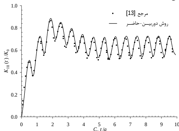
شکل 6 ضریب شدت تنش دینامیکی بی‌بعد، K_{III}(t)/K_0 ، بر حسب زمان بی‌بعد، C_s t/a ، در صفحه بی‌نهایت تحت بار نوسانی با عدد موج \varpi = 5.5 .
