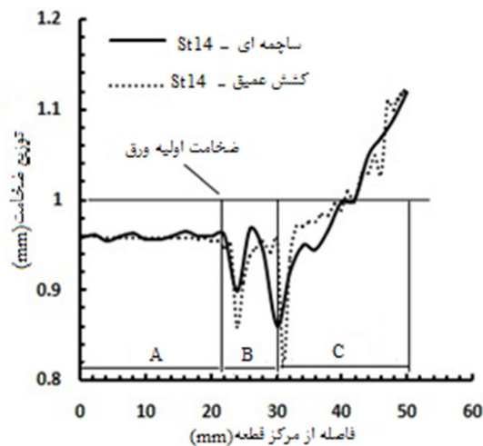
شکل 9 منحنی توزیع ضخامت توسط فرآیندهای ساچمه‌ای و کشش عمیق در شبیه سازی
