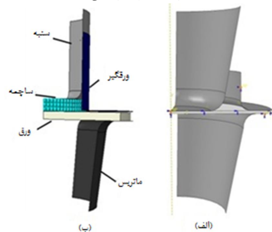
شکل 5 مدل شبیه‌سازی شده الف - کشش عمیق سنتی ب - کشش عمیق ساچمه‌ای
