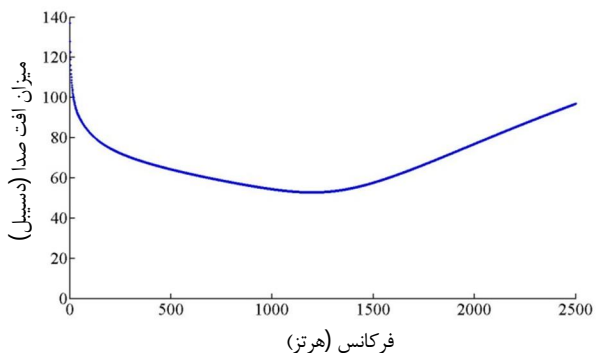
شکل 5 نمودار میزان افت صدا بر حسب فرکانس برای پلی اتیلن (چگالی کم)
