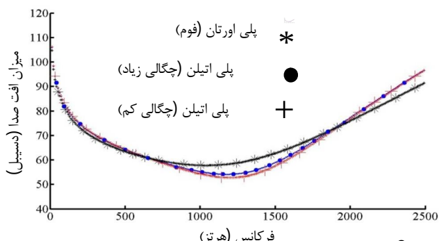
شکل 8 نمودار میزان افت صدا برحسب فرکانس در پوسته دوجداره برای سه جاذب پلی اتیلن (چگالی زیاد)، پلی اتیلن (چگالی کم) و پلی اورتان (فوم)
