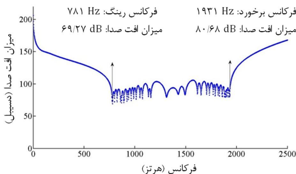
شکل 13 نمودار میزان افت صدا برحسب فرکانس برای گاز هیدروژن
