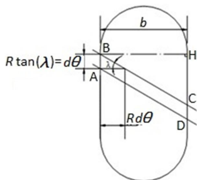
شکل 8 مقطع لوبیایی شکل ورودی بدنه به دریچه
