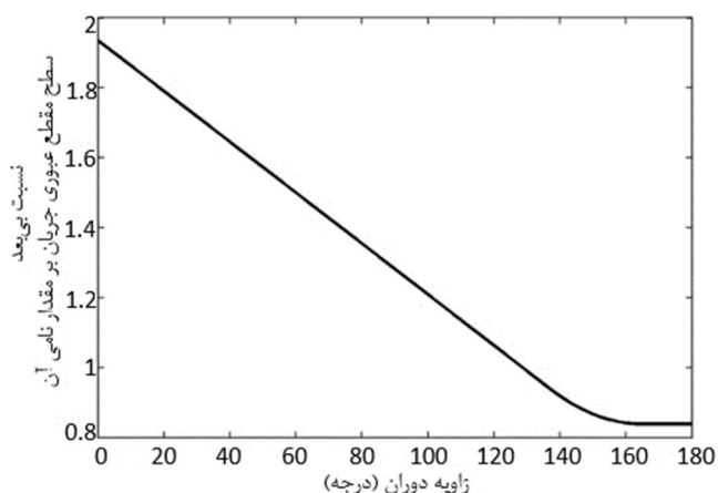
شکل 9 نمودار تغییرات سطح مقطع کنترلی عملگر به‌ازای موقعیت مختلف زاویه‌ای استکانی آن
