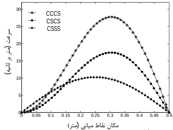
شکل 14 سرعت بیشینه‌ی مرکز ورق برای شرایط مرزی نامتقارن
