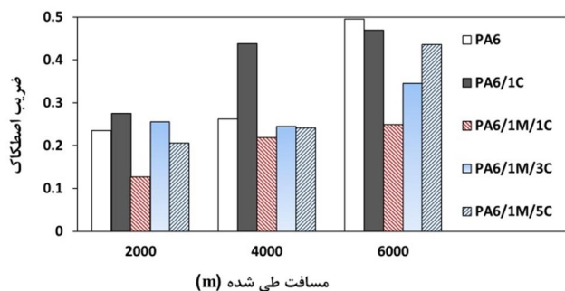
شکل 4 مقایسه‌ی ضریب اصطکاک نمونه‌ها در آزمون سایش
