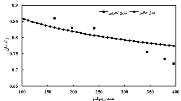
شکل 9 مقایسه نتایج حل عددی حاضر مربوط به سرمایش تبخیری مستقیم با نتایج آزمایشگاهی مرجع [4]
