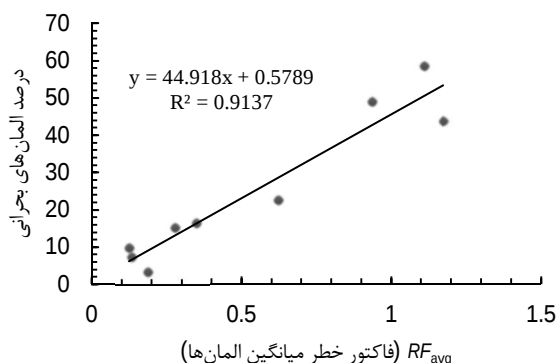
شکل 5 نمودار رابطه‌ی فاکتور خطر با درصد المان‌های بحرانی برای نیروی 9 کیلو نیوتن
