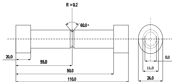
شکل 1 هندسه نمونه‌های RNB (ابعاد به میلی‌متر است) [25].
