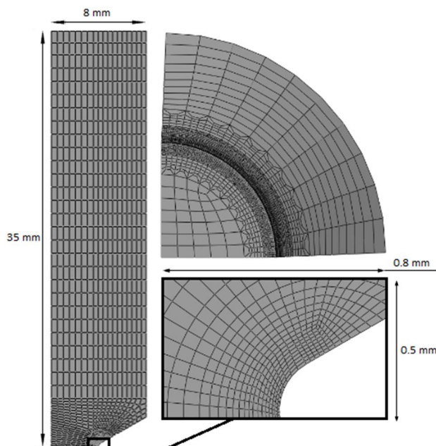
شکل 6 نمایش مش‌بندی مدل سه‌بعدی RNB و المان‌های نزدیک به نوک ترک.
