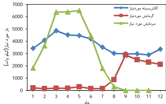
شکل 2 منحنی بار ماهانه الکتریسیته، گرمایش و سرمایه‌های هتل
