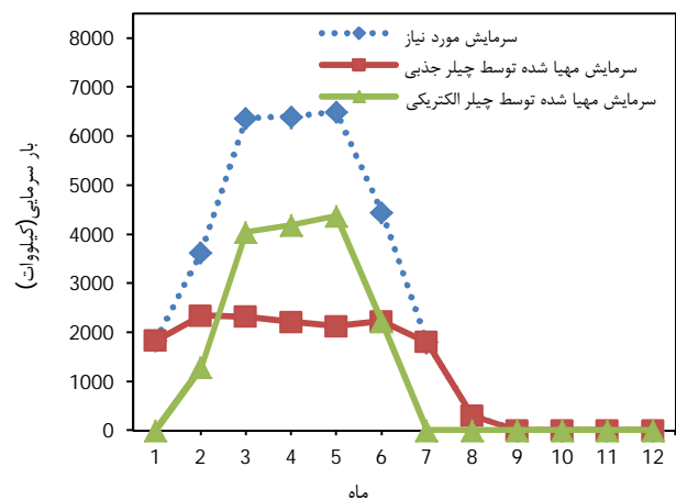
شکل 6 بار سرمایش مهيا شده توسط چيلر جذبي و الكتريكي
